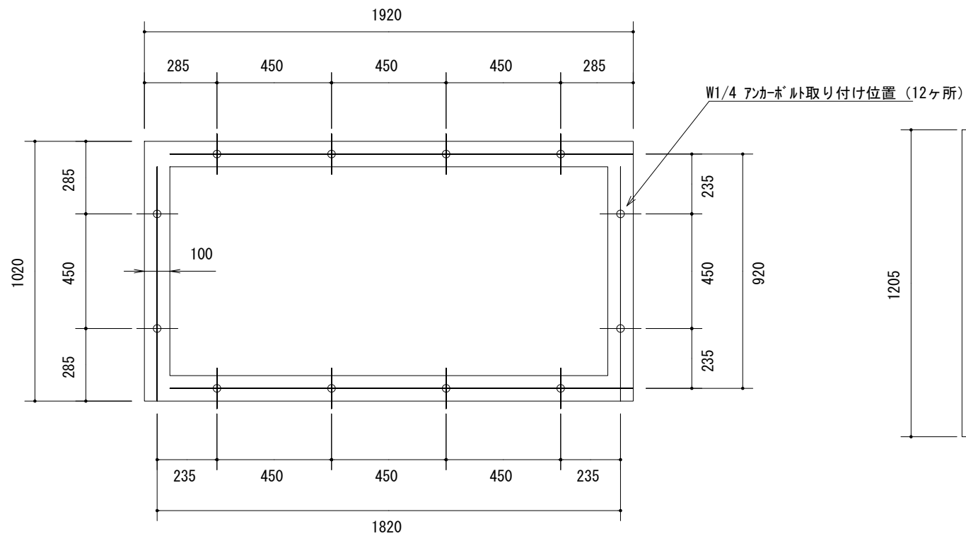
基礎図
